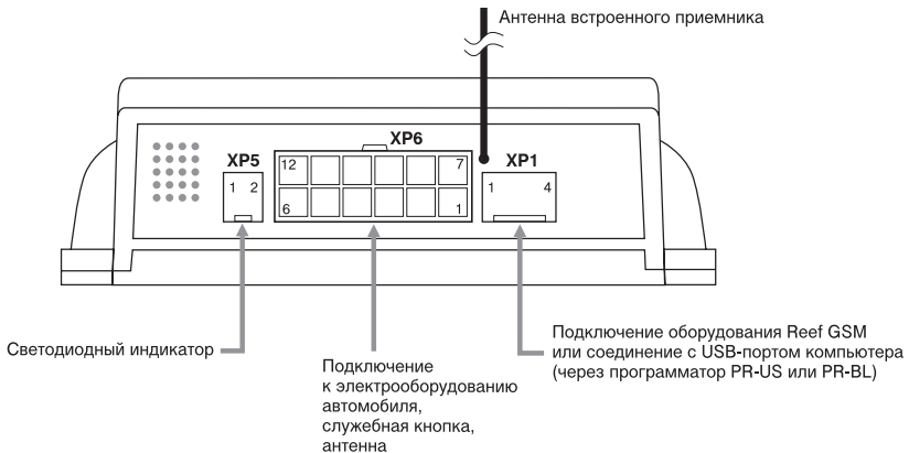
Рис. 1. Назначение разъемов блока управления
