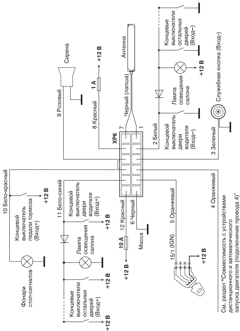
Рис. 2. Подключение к разъему XR6 блока управления
