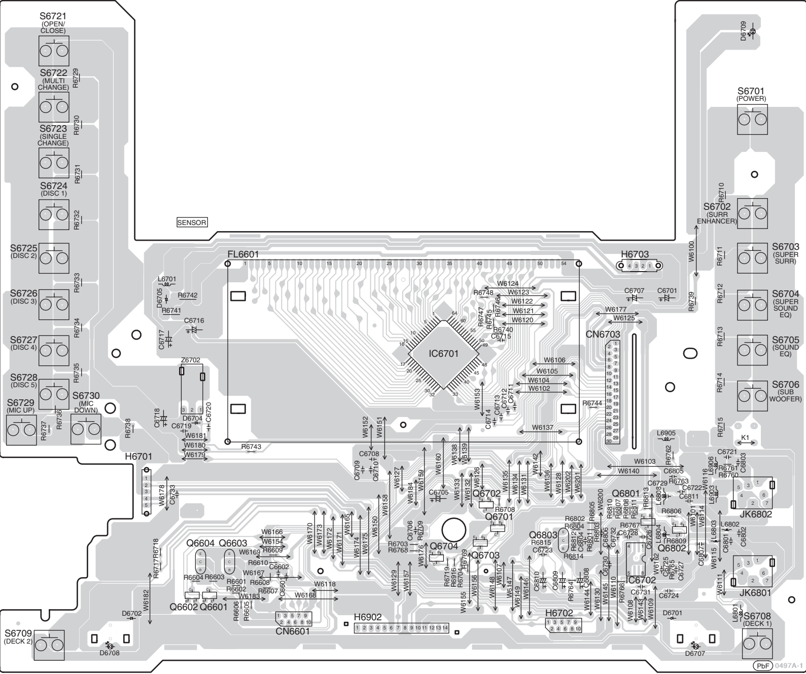
C PANEL P.C.B (REPX0546A)
