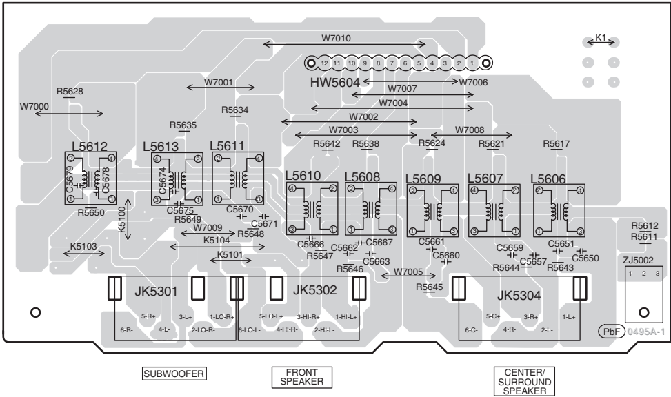
G SPEAKER P.C.B (REPX0544A)
