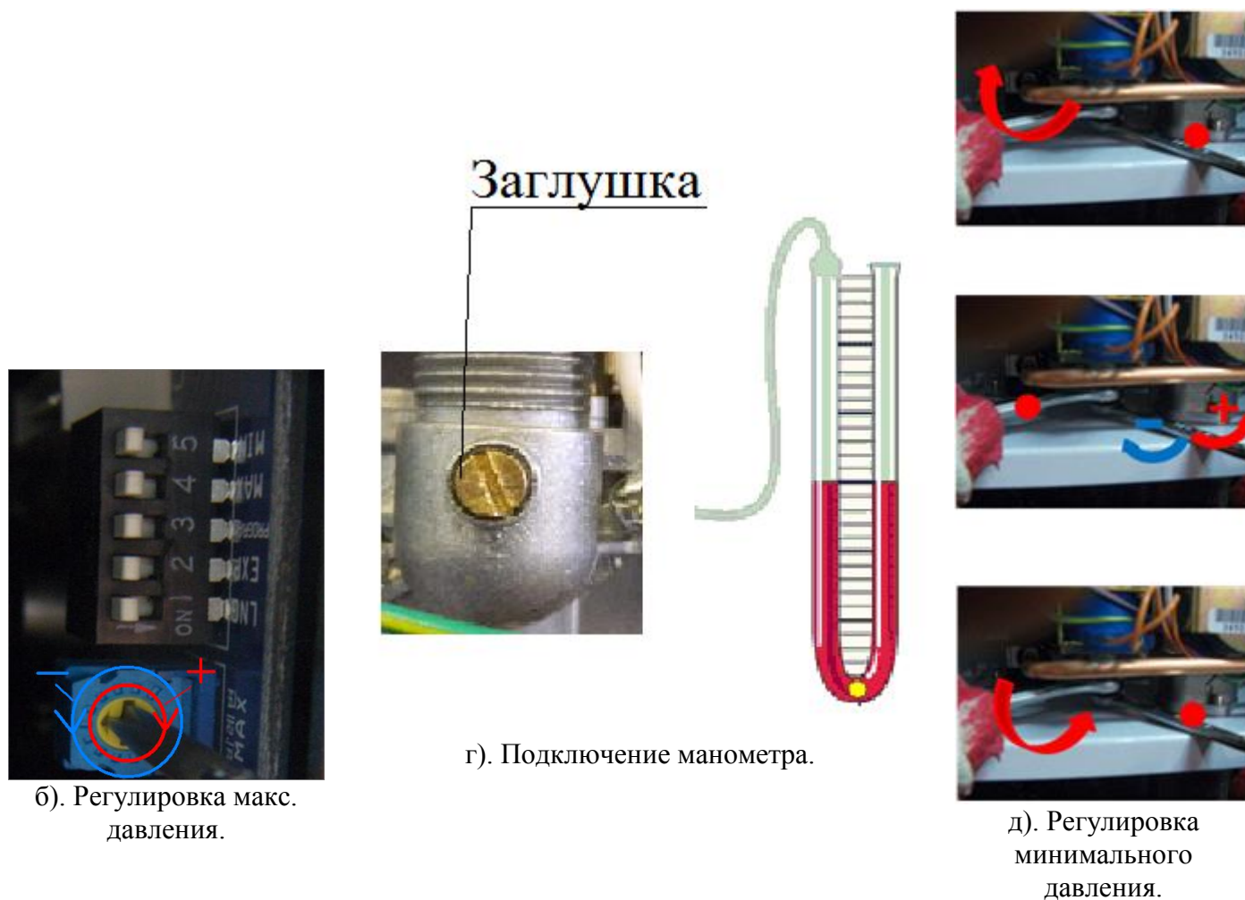
Рис. 9. Регулировка давления газа
